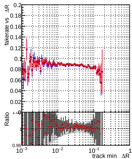
—•— DQM_test_CKFFitDefault —•— DQM_test_doubleFit
