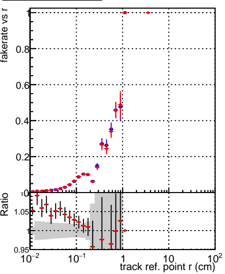
—●— DQM_test_CKFFitDefault —●— DQM_test_doubleFit
