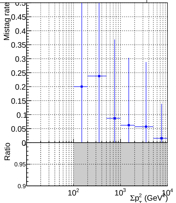
DQM_test_doubleFit
