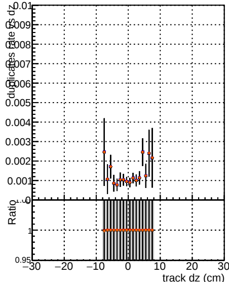
CMSSW-nt08-all7
