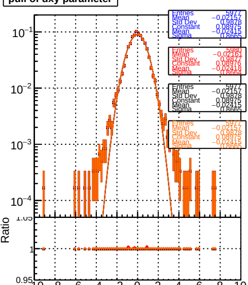
pull of dxy parameter
