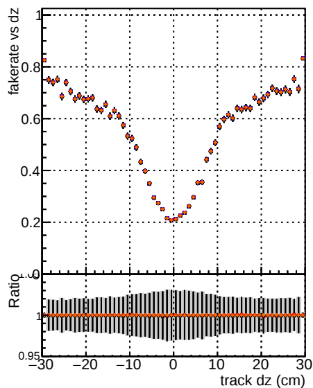
Fake rate vs d d DGM V0001 DGM V0001 P00000000001 Global CMGSW orig Global CMGSW orig Z Global CMSSW dr08 Global CMSSW dr08 Z 0 0.00 0.00 0.00 0.00 0.00 0.00 1 0.00 0.00 0.00 0.00 0.00 0.00 2 0.00 0.00 0.00 0.00 0.00 0.00 3 0.00 0.00 0.00 0.00 0.00 0.00 4 0.00 0.00 0.00 0.00 0.00 0.00 5 0.00 0.00 0.00 0.00 0.00 0.00 6 0.00 0.00 0.00 0.00 0.00 0.00 7 0.00 0.00 0.00 0.00 0.00 0.00 8 0.00 0.00 0.00 0.00 0.00 0.00 9 0.00 0.00 0.00 0.00 0.00 0.00 10 0.00 0.00 0.00 0.00 0.00 0.00
