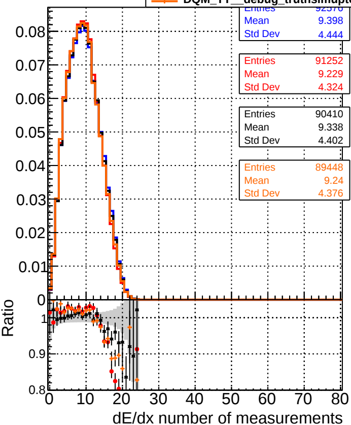
—●— DQM_TT_original —●— DQM_TT_debug_bestinlayer75_epcoh10 —●— DQM_TT_debug_truthallhits75_epcoh11 —●— DQM_TT_debug_truthsimuplayer75_epcoh11
