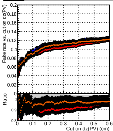
—●— DQM_TT_debug_truthallhits75_epcoh11 —●— DQM_TT_debug_truthsimuptolayer75_epcoh11
