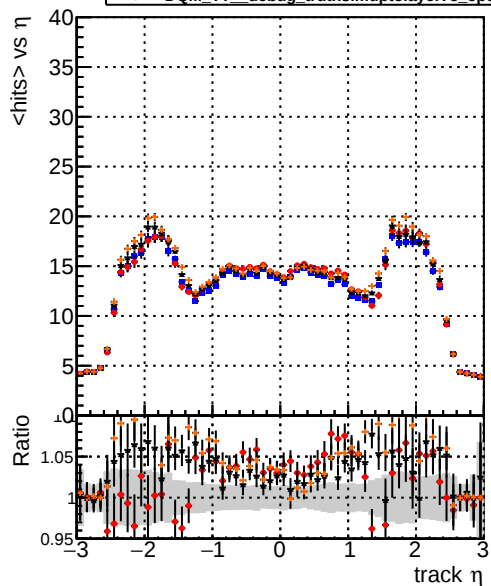
DQM TT original DQM TT debug_bestinlayer75_epcoh10 DQM TT debug_truthallhits75_epcoh11 DQM TT debug_truthsimuptolayer75_epcoh11
