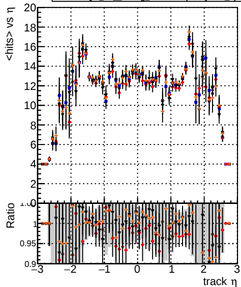
mean hit DQM TT original DQM TT debug_bestinlayer75_epcoh10 DQM TT debug_truthallhits75_epcoh11 DQM TT debug_truthsimuptolayer75_epcoh11
