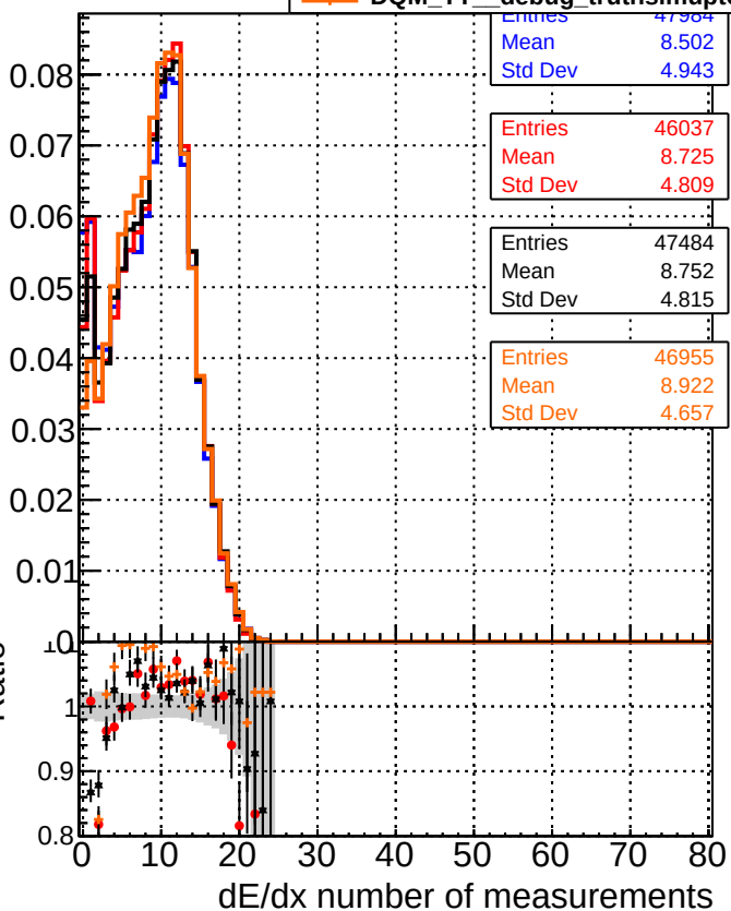
— DQM TT original — DQM TT debug bestinlayer75_epcoh10 — DQM TT debug truthallhits75_epcoh11 — DQM TT debug truthsimptolayer75_epcoh11
