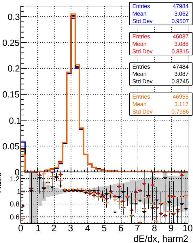
— DQM TT original — DQM TT debug bestinlayer75_epcoh10 — DQM TT debug truthallhits75_epcoh11 — DQM TT debug truthsimptolayer75_epcoh11
