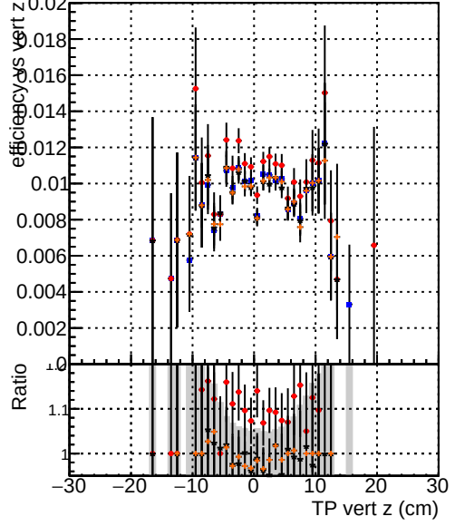
Efficiency vs. TP vert z —●— DQM TT original —●— DQM TT debug_bestinlayer75_epcoh10 —●— DQM TT debug_truthallhits75_epcoh11 —●— DQM TT debug_truthsimuptolayer75_epcoh11
