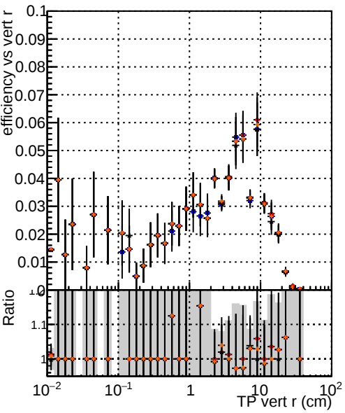
Efficiency vs vertpos —●— DQM TT original_noPU —●— DQM TT paretofrontMaxEffOnlyFWD2_PU —●— DQM TT paretofrontMinFROOnlyFWD2_PU —●— DQM TT paretofrontMaxHitsOnlyFWD2_PU
