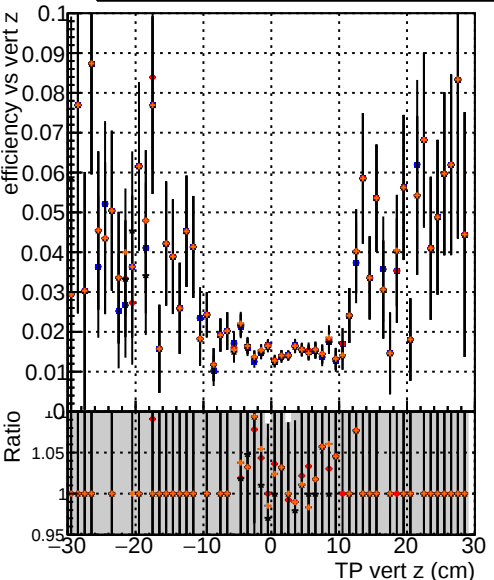
Efficiency vs vertpos —●— DQM TT original_noPU —●— DQM TT paretofrontMaxEffOnlyFWD2_PU —●— DQM TT paretofrontMinFROOnlyFWD2_PU —●— DQM TT paretofrontMaxHitsOnlyFWD2_PU
