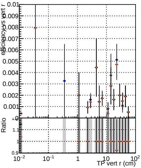
Efficiency vs TP vert r (cm) DQM TT original noPU DQM TT paretofrontMaxEffOnlyFWD2_PU DQM TT paretofrontMinFROnlyFWD2_PU DQM TT paretofrontMaxHitsOnlyFWD2_PU
