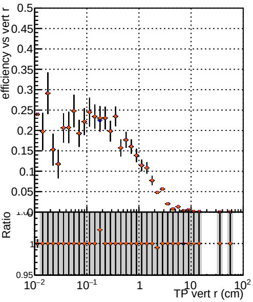
Efficiency vs vertpos —●— DQM TT original noPU —●— DQM TT paretofrontMaxEffOnlyFWD2_PU —●— DQM TT paretofrontMinFROnlyFWD2_PU —●— DQM TT paretofrontMaxHitsOnlyFWD2_PU
