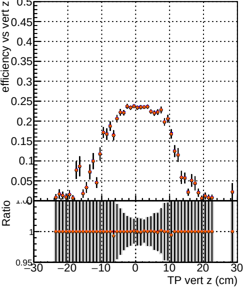
Efficiency vs vertpos —●— DQM TT original noPU —●— DQM TT paretofrontMaxEffOnlyFWD2_PU —●— DQM TT paretofrontMinFROnlyFWD2_PU —●— DQM TT paretofrontMaxHitsOnlyFWD2_PU
