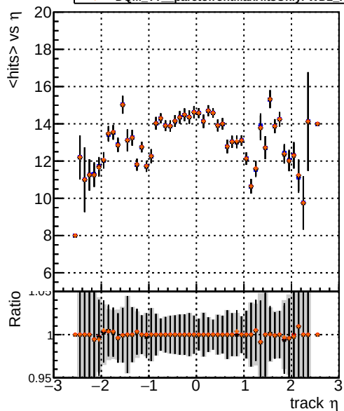
mean hits DQM TT original noPU DQM TT paretofrontMaxEffOnlyFWD2_PU DQM TT paretofrontMinFWD2_PU DQM TT paretofrontMaxHitsOnlyFWD2_PU
