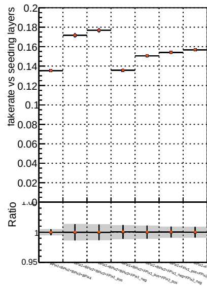
Fake rate vs. BSM IT original noPU BSM IT MaxEffonlFW2 PU BSM IT MaxEffonlFW2 PU
