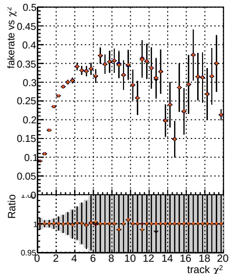
Fake rate vs. BSM IT original noPU BSM IT MaxEffonlFW2 PU BSM IT MaxEffonlFW2 PU
