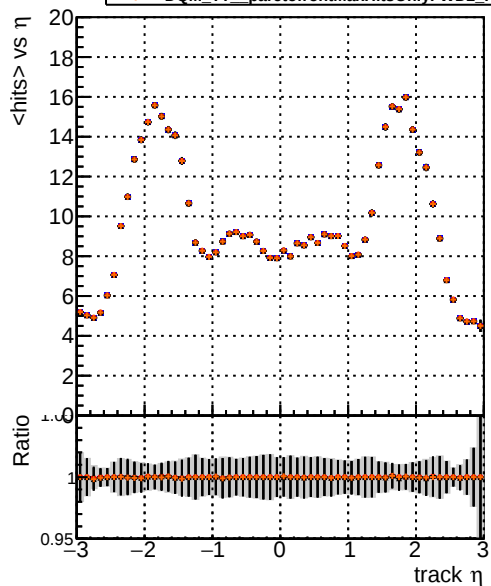
mean hits DQM TT original noPU DQM TT paretofrontMaxEffOnlyFWD2_PU DQM TT paretofrontMinHitsOnlyFWD2_PU DQM TT paretofrontMaxHitsOnlyFWD2_PU
