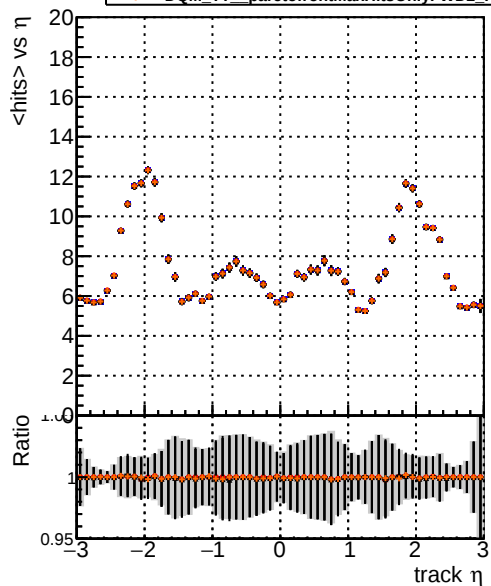
mean hit DQM TT original noPU DQM TT paretofrontMaxEffOnlyFWD2_PU DQM TT paretofrontMinFWD2_PU DQM TT paretofrontMaxHitsOnlyFWD2_PU
