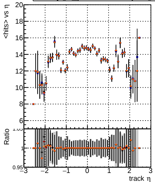
mean hits DQM TT original noPU DQM TT paretofrontMaxEffOnlyFWD2_PU DQM TT paretofrontMinFwdOnlyFWD2_PU DQM TT paretofrontMaxHitsOnlyFWD2_PU
