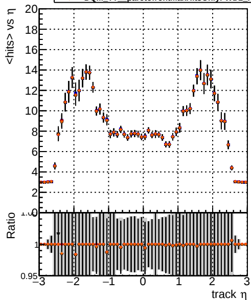
mean hits vs \eta DQM TT original noPU DQM TT paretofrontMaxEffOnlyFWD2_PU DQM TT paretofrontMinFROnlyFWD2_PU DQM TT paretofrontMaxHitsOnlyFWD2_PU
