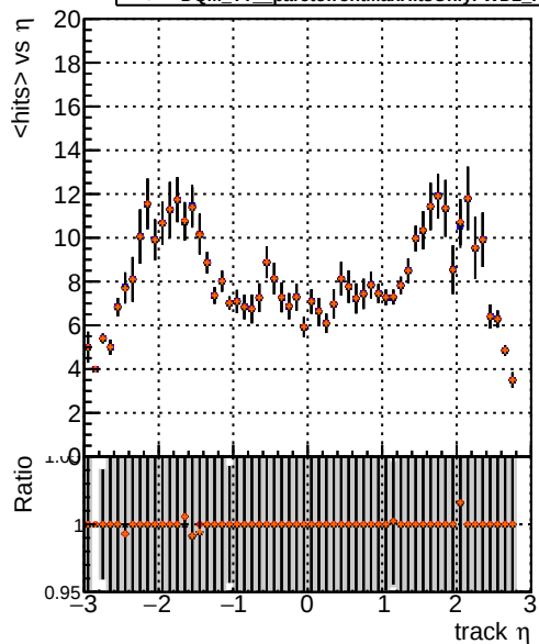
mean hits DQM TT original noPU DQM TT paretofrontMaxEffOnlyFWD2_PU DQM TT paretofrontMinFROnlyFWD2_PU DQM TT paretofrontMaxHitsOnlyFWD2_PU
