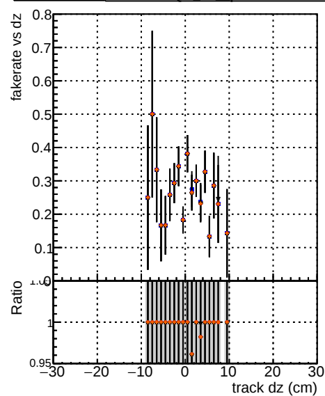
Fake rate vs dz BGM IT original noPU BGM IT BGM IT MaxEffonFWD2 PU BGM IT BGM IT MaxEffonFWD2 PU
