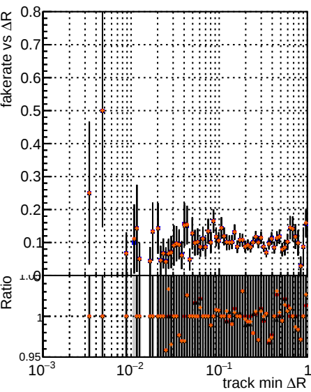
Fake rate vs \Delta R(\text{track, jet}) DQM TT original noPU DQM TT original MaxEffOnlyFWD2_PU DQM TT original MinEffOnlyFWD2_PU DQM TT original HitOnlyFWD2_PU DQM TT original MaxHitOnlyFWD2_PU
