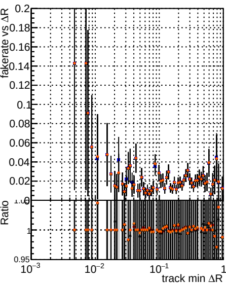
Fake rate vs \Delta R(\text{track}, \text{jet}) Legend: DOM TT original no PU DOM TT paretofrontMinEffOnlyFWD2 PU DOM TT paretofrontMinHitOnlyFWD2 PU DOM TT paretofrontMaxHitOnlyFWD2 PU
