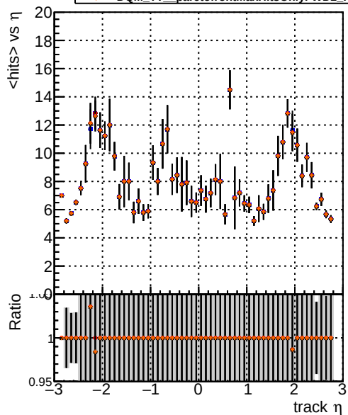
mean hit DQM TT original noPU DQM TT paretofrontMaxEffOnlyFWD2_PU DQM TT paretofrontMinFROnlyFWD2_PU DQM TT paretofrontMaxHitsOnlyFWD2_PU
