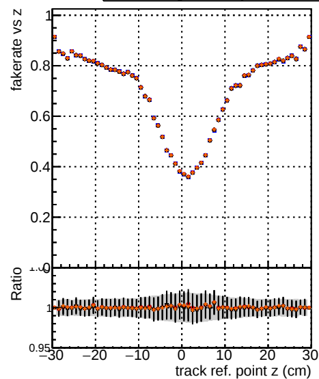
DOM TT original no PU DOM TT paretofrontMaxEffOnlyFWD2 PU DOM TT paretofrontMinEffOnlyFWD2 PU DOM TT paretofrontMaxHitOnlyFWD2 PU
