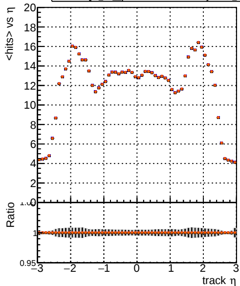
DQM TT original noPU DQM TT paretofrontMaxEffOnlyFWD2_PU DQM TT paretofrontMinFROnlyFWD2_PU DQM TT paretofrontMaxHitsOnlyFWD2_PU
