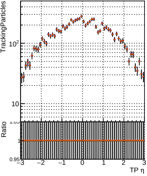
—●— DQM TT original noPU —●— DQM TT paretofrontMaxEffOnlyFWD2_PU —●— DQM TT paretofrontMinFROnlyFWD2_PU —●— DQM TT paretofrontMaxHitsOnlyFWD2_PU
