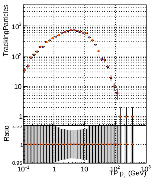
— DQM TT original_noPU — DQM TT paretofrontMaxEffOnlyFWD2_PU — DQM TT paretofrontMinFROOnlyFWD2_PU — DQM TT paretofrontMaxHitsOnlyFWD2_PU
