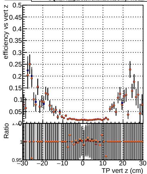
Efficiency vs. TP vert z —●— DQM TT original noPU —●— DQM TT paretofrontMaxEffOnlyFWD2_PU —●— DQM TT paretofrontMinFROOnlyFWD2_PU —●— DQM TT paretofrontMaxHitsOnlyFWD2_PU
