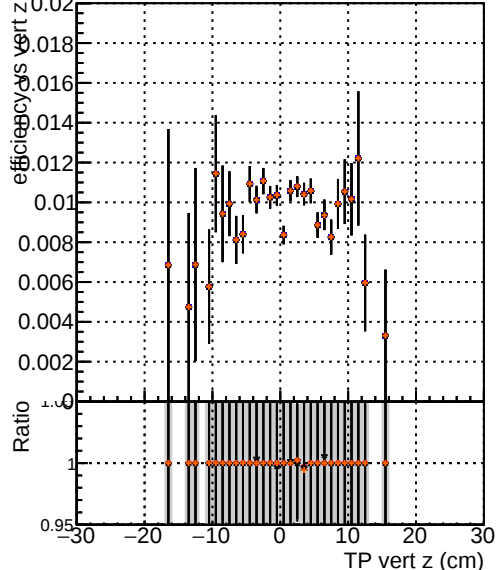
Efficiency vs. TP vert z —●— DQM TT original noPU —●— DQM TT paretofrontMaxEffOnlyFWD2_PU —●— DQM TT paretofrontMinFROnlyFWD2_PU —●— DQM TT paretofrontMaxHitsOnlyFWD2_PU
