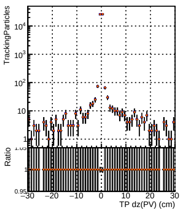
N of simulated tracks vs dz(PV) 1000 2000 3000 4000 5000 6000 7000 8000 9000 10000 11000 12000 13000 14000 15000 16000 17000 18000 19000 20000 21000 22000 23000 24000 25000 26000 27000 28000 29000 30000 31000 32000 33000 34000 35000 36000 37000 38000 39000 40000 41000 42000 43000 44000 45000 46000 47000 48000 49000 50000 51000 52000 53000 54000 55000 56000 57000 58000 59000 60000 61000 62000 63000 64000 65000 66000 67000 68000 69000 70000 71000 72000 73000 74000 75000 76000 77000 78000 79000 80000 81000 82000 83000 84000 85000 86000 87000 88000 89000 90000 91000 92000 93000 94000 95000 96000 97000 98000 99000 100000
