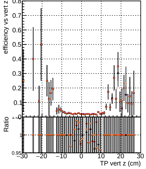
Efficiency vs vert z —●— DQM TT original noPU —●— DQM TT paretofrontMaxEffOnlyFWD2_PU —●— DQM TT paretofrontMinFROOnlyFWD2_PU —●— DQM TT paretofrontMaxHitsOnlyFWD2_PU
