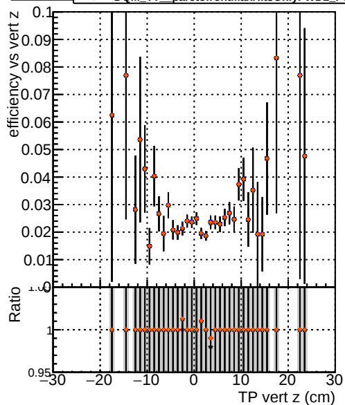
Efficiency vs vert z —●— DQM TT original_noPU —●— DQM TT paretofrontMaxEffOnlyFWD2_PU —●— DQM TT paretofrontMinFROnlyFWD2_PU —●— DQM TT paretofrontMaxHitsOnlyFWD2_PU
