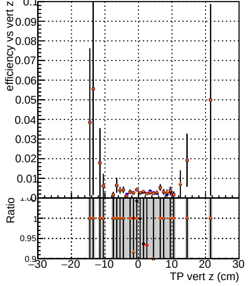
Efficiency vs. TP vert z (cm) —●— DQM TT original noPU —●— DQM TT paretofrontMaxEffOnlyFWD2_PU —●— DQM TT paretofrontMinFROOnlyFWD2_PU —●— DQM TT paretofrontMaxHitsOnlyFWD2_PU
