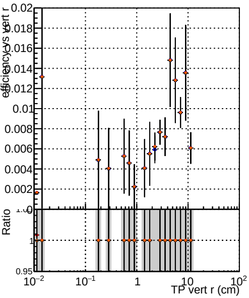
Efficiency vs TP vert r (cm) DQM TT original noPU DQM TT paretofrontMaxEffOnlyFWD_PU DQM TT paretofrontMinFROnlyFWD_PU DQM TT paretofrontMaxHitsOnlyFWD_PU
