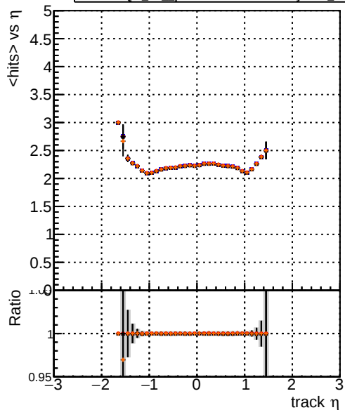
mean hit DQM TT original noPU DQM TT paretofrontMaxEffOnlyFWD_PU DQM TT paretofrontMinFOnlyFWD_PU DQM TT paretofrontMaxHitsOnlyFWD_PU
