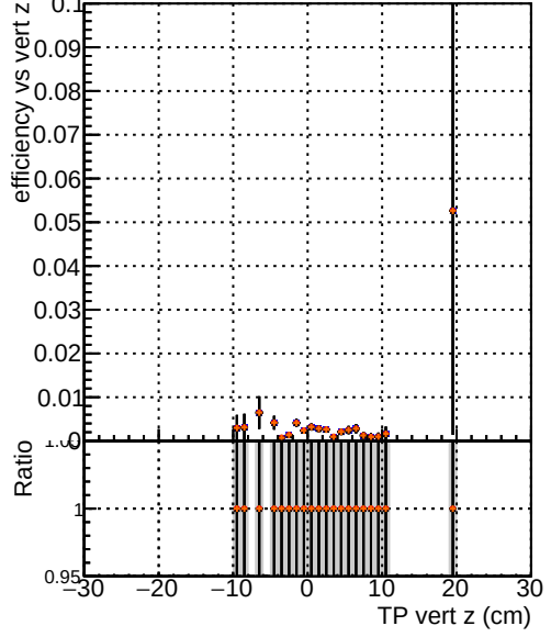
Efficiency vs TP vert z —●— DQM TT original noPU —●— DQM TT paretofrontMaxEffOnlyFWD_PU —●— DQM TT paretofrontMinFROnlyFWD_PU —●— DQM TT paretofrontMaxHitsOnlyFWD_PU
