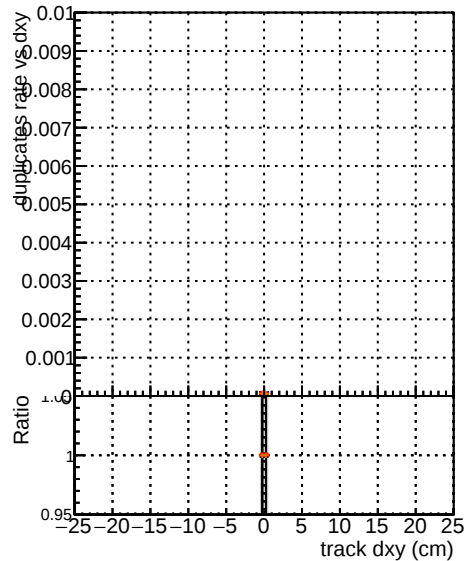
Only use these tags: ['math>, \frac{1}{2} , \frac{1}{4} , \frac{1}{8} , \frac{1}{16} , \frac{1}{32} , \frac{1}{64} , \frac{1}{128} , \frac{1}{256} , \frac{1}{512} , \frac{1}{1024} , \frac{1}{2048} , \frac{1}{4096} , \frac{1}{8192} , \frac{1}{16384} , \frac{1}{32768} , \frac{1}{65536} , \frac{1}{131072} , \frac{1}{262144} , \frac{1}{524288} , \frac{1}{1048576} , \frac{1}{2097152} , \frac{1}{4194304} , \frac{1}{8388608} , \frac{1}{16777216} , \frac{1}{33554432} , \frac{1}{67108864} , \frac{1}{134217728} , \frac{1}{268435456} , \frac{1}{536870912} , \frac{1}{1073741824} , \frac{1}{2147483648} , \frac{1}{4294967296} , \frac{1}{8589934592} , \frac{1}{17179869184} , \frac{1}{34359738368} , \frac{1}{68719476736} , \frac{1}{137438953472} , \frac{1}{274877906944} , \frac{1}{549755813888} , \frac{1}{1099511627776} , \frac{1}{2199023255552} , \frac{1}{4398046511104} , \frac{1}{8796093022208} , \frac{1}{17592186044416} , \frac{1}{35184372088832} , \frac{1}{70368744177664} , \frac{1}{140737488355328} , \frac{1}{281474976710656} , \frac{1}{562949953421312} , \frac{1}{1125899906842624} , \frac{1}{2251799813685248} , \frac{1}{4503599627370496} , \frac{1}{9007199254740992} , \frac{1}{18014398509481984} , \frac{1}{36028797018963968} , \frac{1}{72057594037927936} , \frac{1}{144115188075855872} , \frac{1}{288230376151711744} , \frac{1}{576460752303423488} , \frac{1}{1152921504606846976} , \frac{1}{2305843009213693952} , \frac{1}{4611686018427387904} , \frac{1}{9223372036854775808} , \frac{1}{18446744073709551616} , \frac{1}{36893488147419103232} , \frac{1}{73786976294838206464} , \frac{1}{147573952589676412928} , \frac{1}{295147905179352825856} , \frac{1}{590295810358705651712} , \frac{1}{1180591620717411303424} , \frac{1}{2361183241434822606848} , \frac{1}{4722366482869645213696} , \frac{1}{9444732965739290427392} , \frac{1}{18889465931478580854784} , \frac{1}{37778931862957161709568} , \frac{1}{75557863725914323419136} , \frac{1}{151115727451828646838272} , \frac{1}{302231454903657293676544} , \frac{1}{604462909807314587353088} , \frac{1}{1208925819614629174706176} , \frac{1}{2417851639229258349412352} , \frac{1}{4835703278458516698824704} , \frac{1}{9671406556917033397649408} , \frac{1}{19342813113834066795298816} , \frac{1}{38685626227668133590597632} , \frac{1}{77371252455336267181195264} , \frac{1}{154742504910672534362390528} , \frac{1}{309485009821345068724781056} , \frac{1}{618970019642690137449562112} , \frac{1}{1237940039285380274899124224} , \frac{1}{2475880078570760549798248448} , \frac{1}{4951760157141521099596496896} , \frac{1}{9903520314283042199192993792} , \frac{1}{19807040628566084398385987584} , \frac{1}{39614081257132168796771975168} , \frac{1}{79228162514264337593543950336} , \frac{1}{158456325028528675187087900672} , \frac{1}{316912650057057350374175801344} , \frac{1}{633825300114114700748351602688} , \frac{1}{1267650600228229401496703205376} , \frac{1}{2535301200456458802993406410752} , \frac{1}{5070602400912917605986812821504} , \frac{1}{10141204801825835211973625643008} , \frac{1}{20282409603651670423947251286016} , \frac{1}{40564819207303340847894502572032} , \frac{1}{81129638414606681695789005144064} , \frac{1}{162259276829213363391578010288128} , \frac{1}{324518553658426726783156020576256} , \frac{1}{649037107316853453566312041152512} , \frac{1}{1298074214633706907132624082305024} , \frac{1}{2596148429267413814265248164610048} , \frac{1}{5192296858534827628530496329220096} , \frac{1}{10384593717069655257060992658440192} , \frac{1}{20769187434139310514121985316880384} , \frac{1}{41538374868278621028243970633760768} , \frac{1}{83076749736557242056487941267521536} , \frac{1}{166153499473114484112975882535043072} , \frac{1}{332306998946228968225951765070086144} , \frac{1}{664613997892457936451903530140172288} , \frac{1}{1329227995784915872903807060280344576} , \frac{1}{2658455991569831745807614120560689152} , \frac{1}{5316911983139663491615228241121378304} , \frac{1}{10633823966279326983230456482242756608} , \frac{1}{21267647932558653966460912964485513216} , \frac{1}{42535295865117307932921825928971026432} , \frac{1}{85070591730234615865843651857942052864} , \frac{1}{170141183460469231731687303715884105728} , \frac{1}{340282366920938463463374607431768211456} , \frac{1}{680564733841876926926749214863536422912} , \frac{1}{1361129467683753853853498429727072845824} , \frac{1}{2722258935367507707706996859454145691648} , \frac{1}{5444517870735015415413993718908291383296} , \frac{1}{10889035741470030830827987437816582766592} , \frac{1}{2
