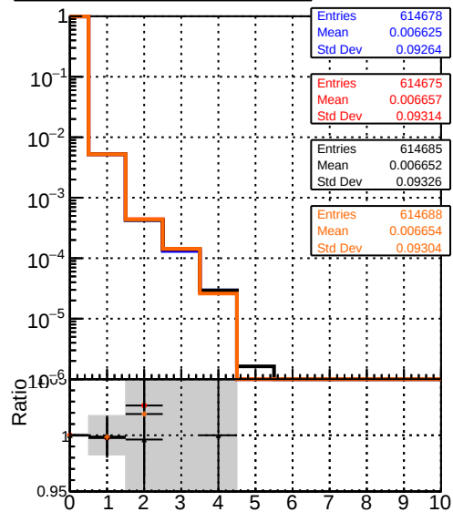
mean hits DQM TT original noPU DQM TT paretofrontMaxEffOnlyFWD_PU DQM TT paretofrontMinFROnlyFWD_PU DQM TT paretofrontMaxHitsOnlyFWD_PU
