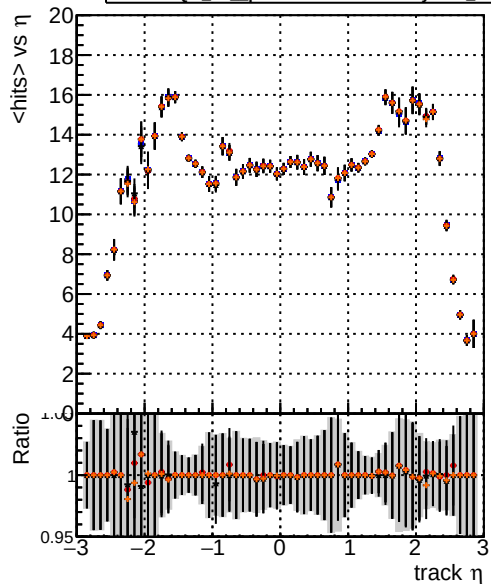
mean hits DQM TT original noPU DQM TT paretofrontMaxEffOnlyFWD_PU DQM TT paretofrontMinFROnlyFWD_PU DQM TT paretofrontMaxHitsOnlyFWD_PU
