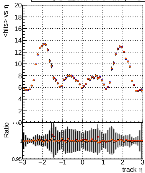
mean hit DQM TT original noPU DQM TT paretofrontMaxEffOnlyFWD_PU DQM TT paretofrontMinFROnlyFWD_PU DQM TT paretofrontMaxHitsOnlyFWD_PU
