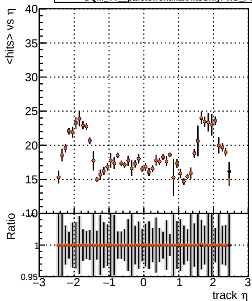
mean hit DQM TT original noPU DQM TT paretofrontMaxEffOnlyFWD_PU DQM TT paretofrontMinFwdOnlyFWD_PU DQM TT paretofrontMaxHitsOnlyFWD_PU
