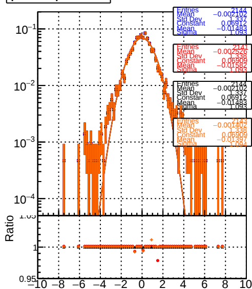
\forall \theta \in \Theta pull of \theta parameter
