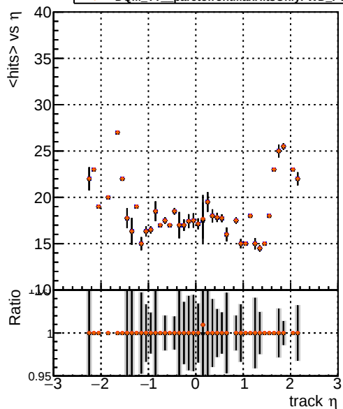
mean hit DQM TT original noPU DQM TT paretofrontMaxEffOnlyFWD_PU DQM TT paretofrontMinFOnlyFWD_PU DQM TT paretofrontMaxHitsOnlyFWD_PU
