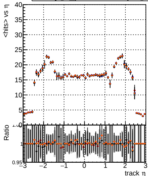
mean hits DQM TT original noPU DQM TT paretofrontMaxEffOnlyFWD_PU DQM TT paretofrontMinFwdOnlyFWD_PU DQM TT paretofrontMaxHitsOnlyFWD_PU
