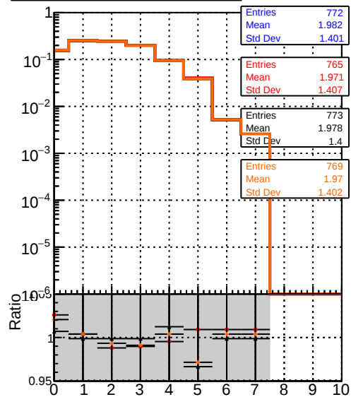
mean hit DQM TT original noPU DQM TT paretofrontMaxEffOnlyFWD_PU DQM TT paretofrontMinFROnlyFWD_PU DQM TT paretofrontMaxHitsOnlyFWD_PU
