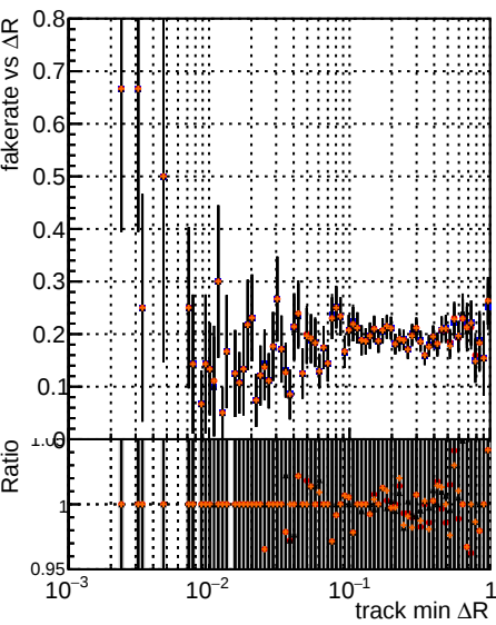
Fake rate vs \Delta R(\text{track, jet}) DQM TT original noPU DQM TT paretofrontMinEffOnlyFWD_PU DQM TT paretofrontMinHitOnlyFWD_PU DQM TT paretofrontMaxHitOnlyFWD_PU
