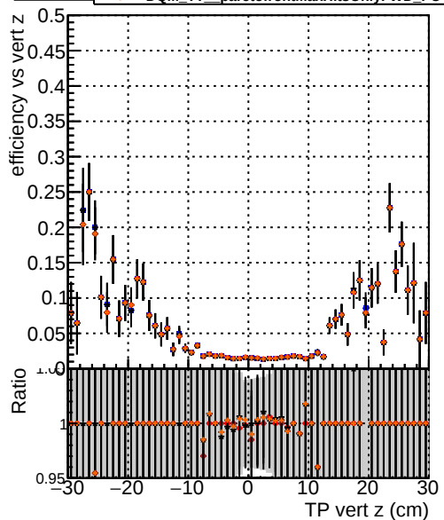
Efficiency vs. TP vert z (cm) —●— DQM TT original noPU —●— DQM TT paretofrontMaxEffOnlyFWD_PU —●— DQM TT paretofrontMinFROnlyFWD_PU —●— DQM TT paretofrontMaxHitsOnlyFWD_PU
